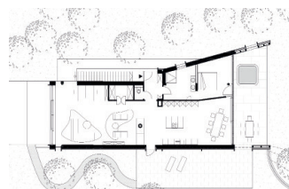
Grundriss Obergeschoß
