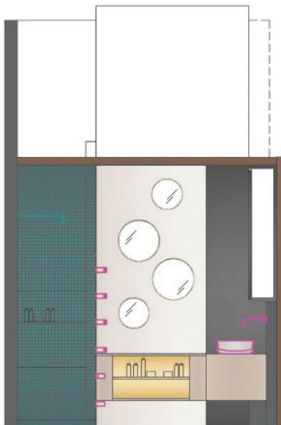
Schnitt
