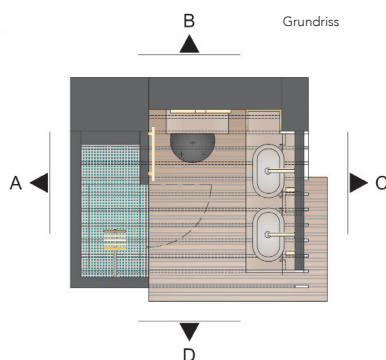
Grundriss
